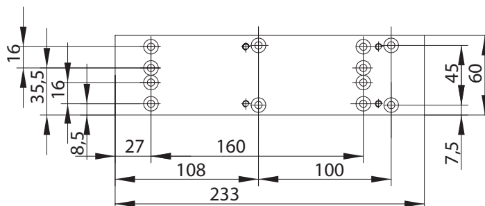
Montageplaat A187
