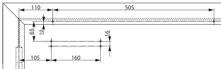
2 - Deurbladmontage niet-scharnierzijde
