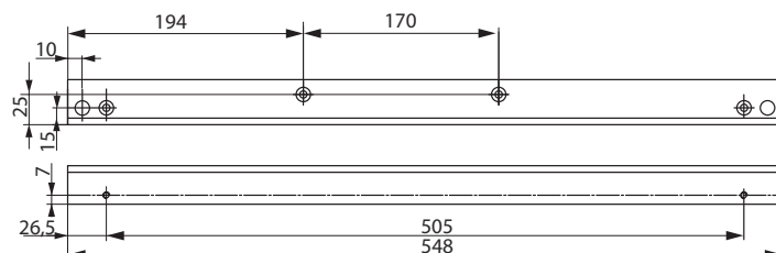
Hoekmontageplaat A116 Voor glijarm G460 op niet-scharnierzijde.
