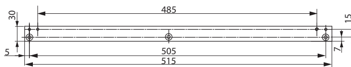
Vlakke montageplaat A115 Voor glijarm G460.
